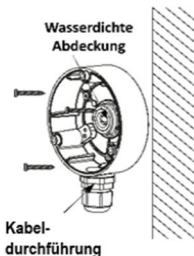
Abbildung 2-6 Befestigung der Anschlussdose an der Wand
