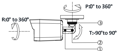
Abbildung 2-3 3-Achsen Einstellung
