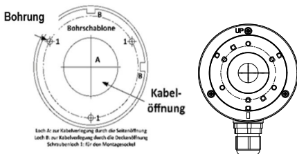
Abbildung 2-4 Bohrschablone
