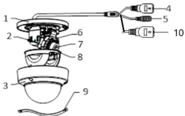
Abbildung 1-1 Kamera Übersicht
