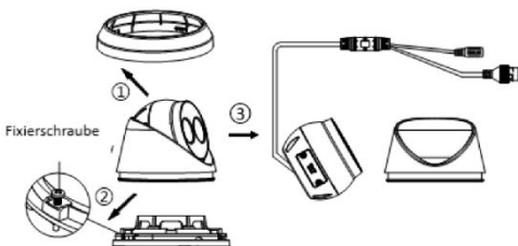
Abbildung 2.2 Zerlegen der Kamera
