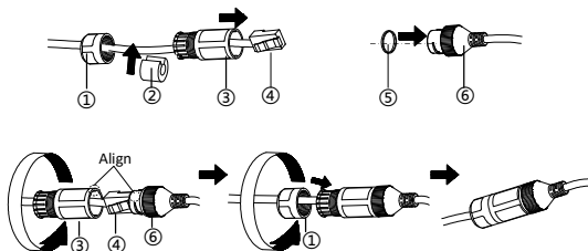
Abbildung 2.8 Installation der wasserdichten Hülle
