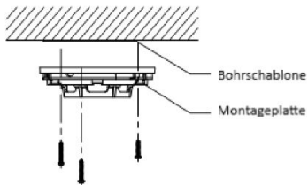
Abbildung 2.4 Montageplatte befestigen
