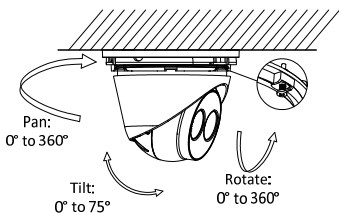
Abbildung 2.6 Blickwinkel einstellen
