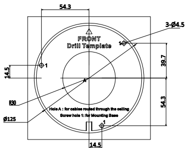
Abbildung 2.3 Bohrschablone
