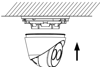
Abbildung 2.5 Installieren der Kamera
