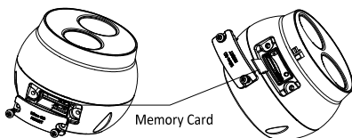
Abbildung 2.1 Abdeckung entfernen
