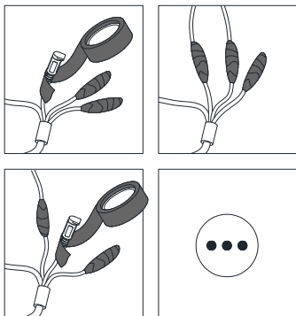
Abbildung 2.9 Kabel Abdichtungen
