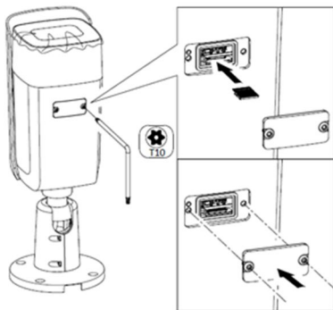
Abbildung 2-1 Speicherkarte einsetzen
