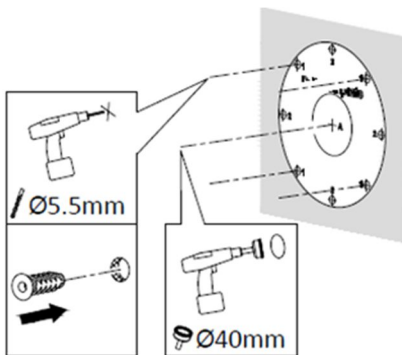
Abbildung 2-2 Bohren Sie Löcher in die Wand / Decke gemäß der Bohrschablone
