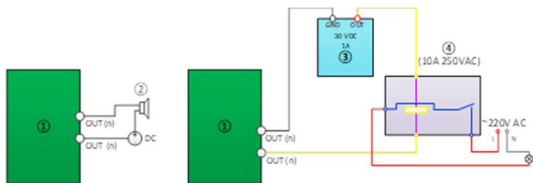
Abbildung 1-3 Alarmausgang
