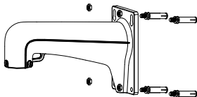
Abbildung 2-4 Wandhalterung anbringen
