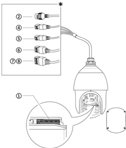
Abbildung 1-2 Kabelübersicht
