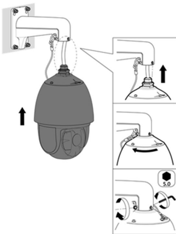
Abbildung 2-6 Sicherheitsseil
