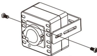
Abbildung 2-2 Kamera befestigen
