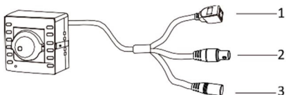
Abbildung 1-1 Kamera Überblick
