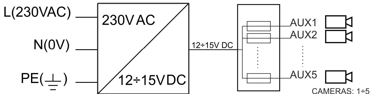
Bild.1. Schaltplan Netzteil.
