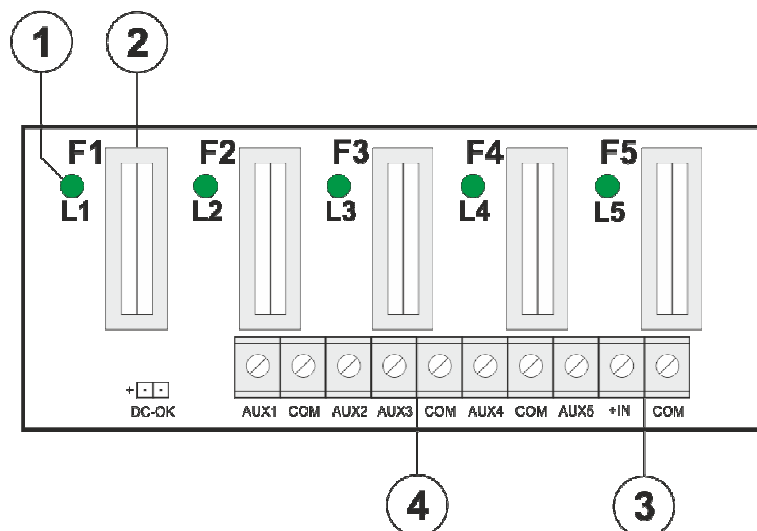
Bild. 2. Blick auf die Netzteilplatte PCB.
