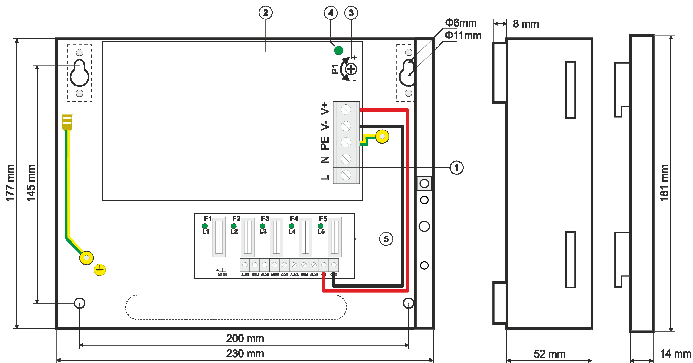
Bild.3. Netzteil-Ansicht.
