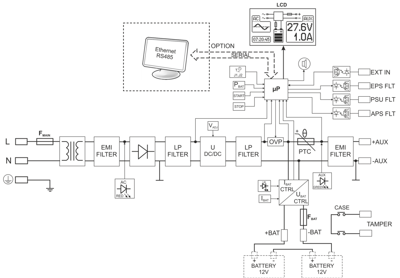
Abb. 1. Das Blockscha des Netzgeräts.
