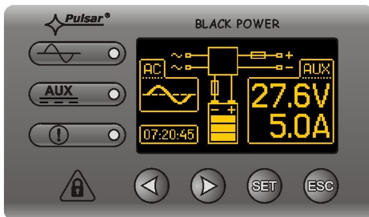
Abb. 5. Kontrollpanel.
