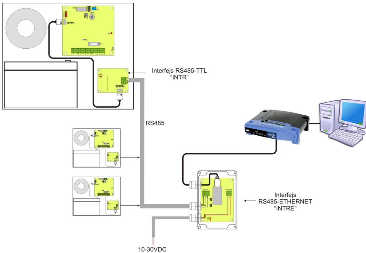
Abb. 26. Komunikation Ethernet mit der Nutzung des Interfaces RS485-Ethernet „INTRE“.
