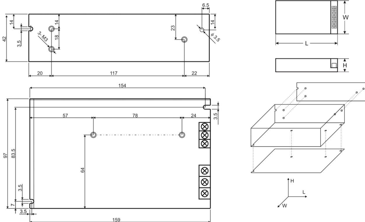
Abbildung 2. Mechanische Ansicht der Speiseleitung.
