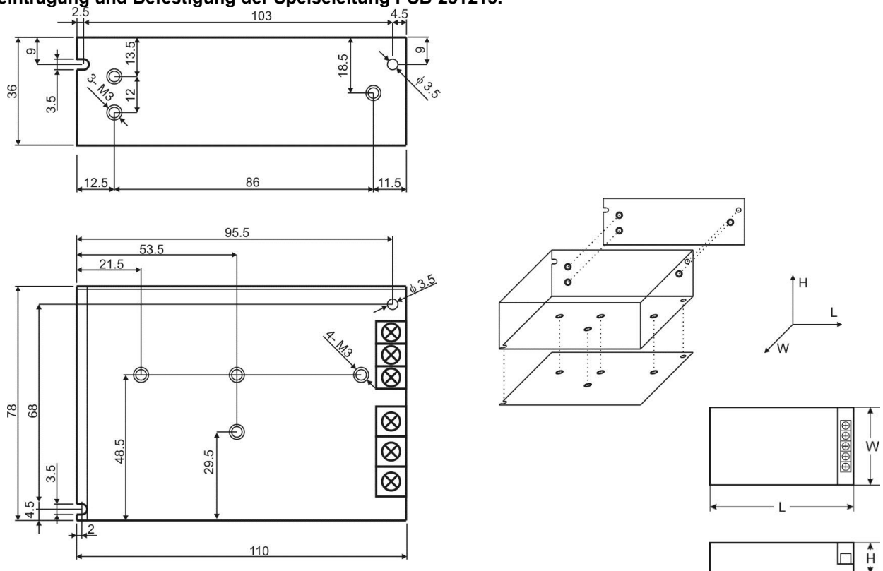
Abbildung 2. Mechanische Ansicht der Speiseleitung.
