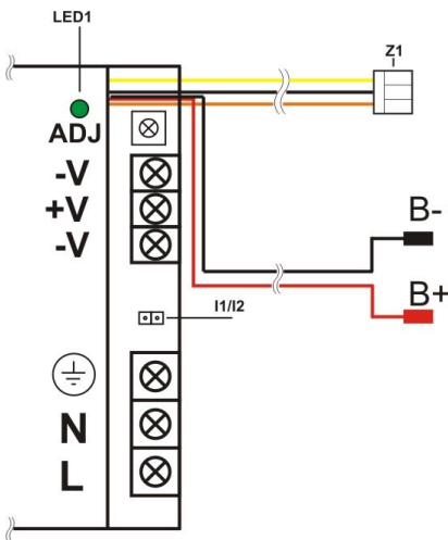
Abbildung 1. Beschreibung der Verbindungsstücke der Speiseleitung.
