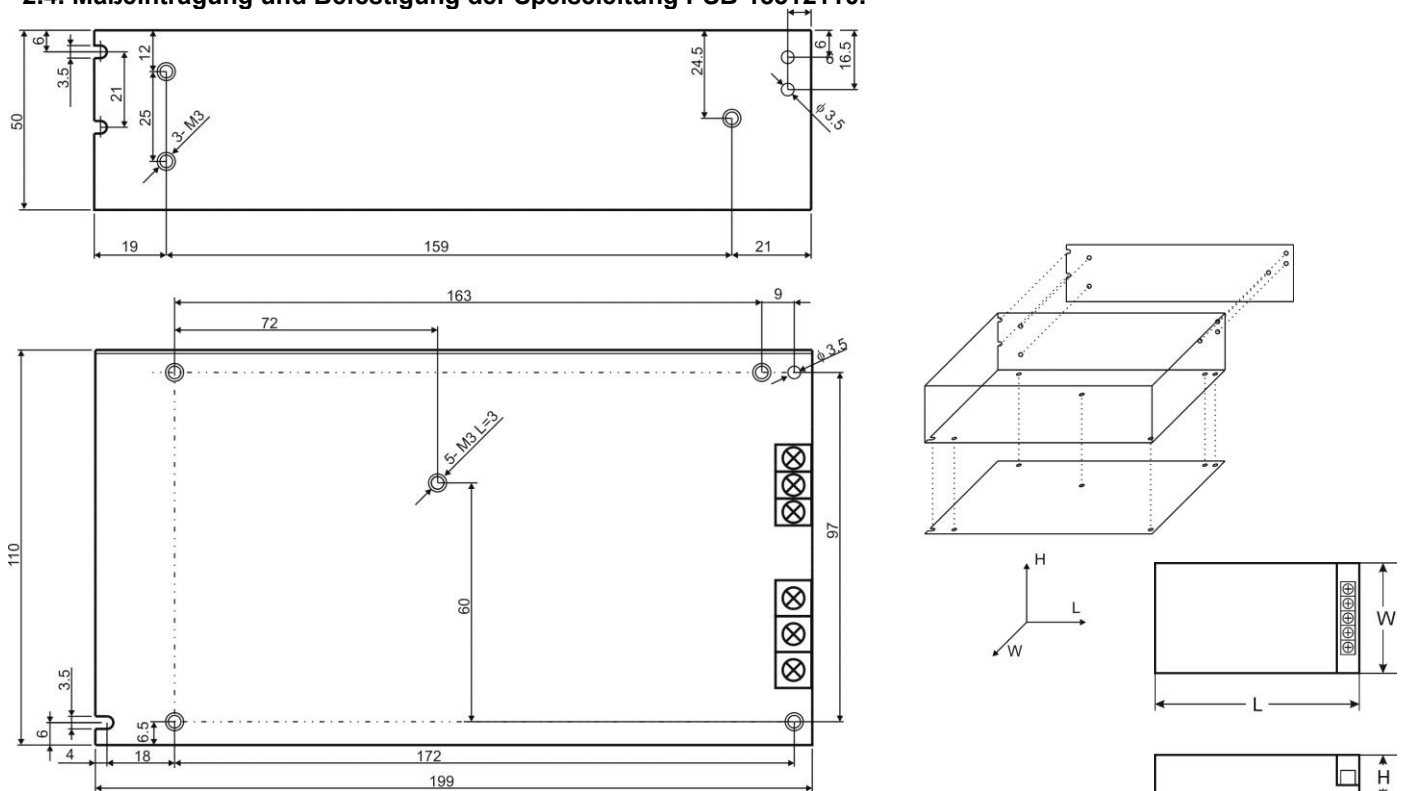
Abbildung 2. Mechanische Ansicht der Speiseleitung.
