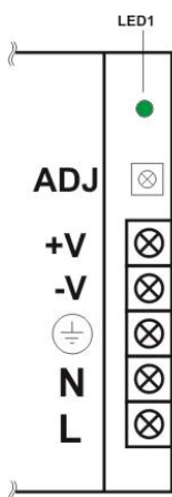
Abbildung 1. Beschreibung der Netzteilstöße.
