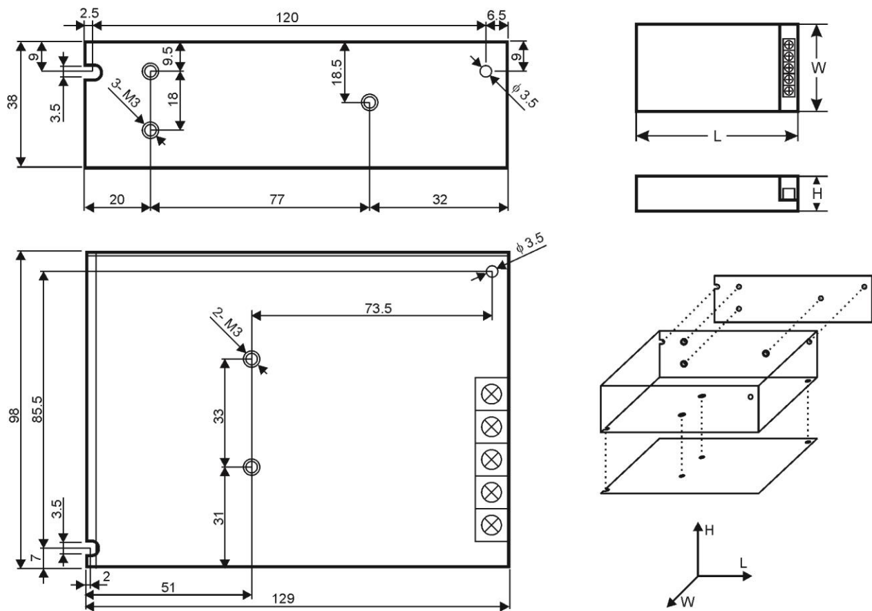
Abbildung 2. Mechanische Ansicht des Netzteil
