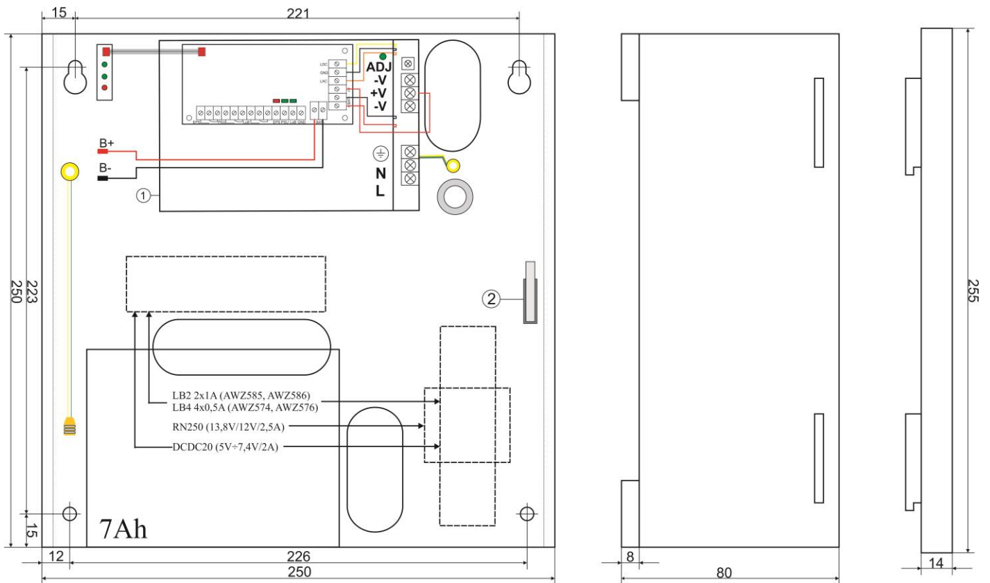
Abb. 3. Ansicht des Netzteils.
