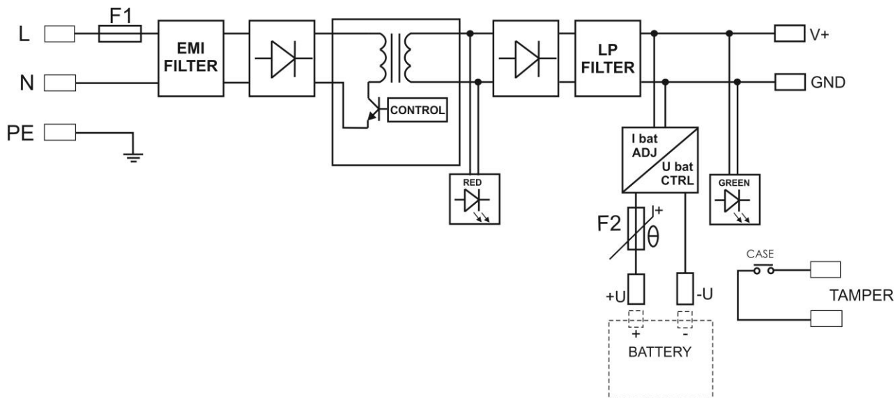
Bild 1. Schaltplan Netzteil.
