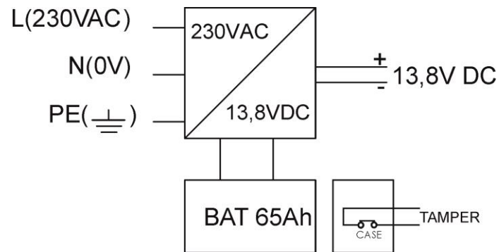
Bild 1. Schaltplan Netzteil.
