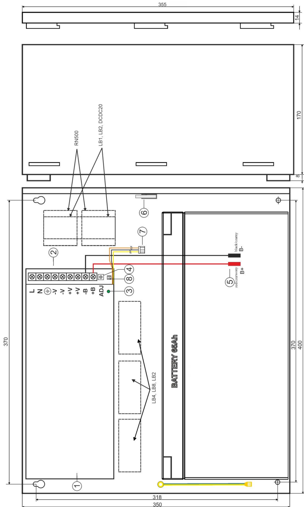
Bild 2. Netzteil-Ansicht.
