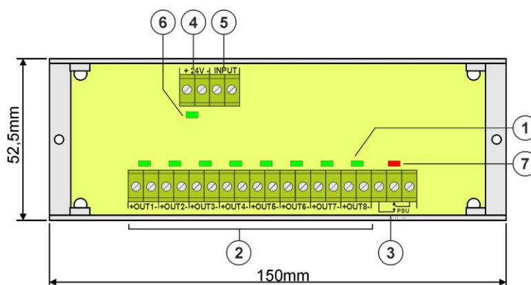
Fig.1. Module view.
