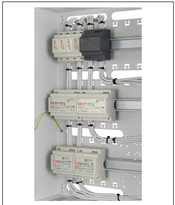
Fig.2 Mounting DIN rails on plastic brackets - 20mm (wyposażenie standardowe)
