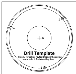
Abbildung 2-1 Bohrschablone
