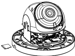
Abbildung 2-2 Speicherkarte einlegen
