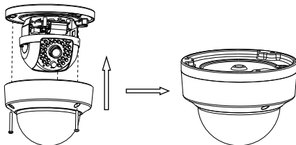
Abbildung 2-8 Kuppel wieder befestigen
