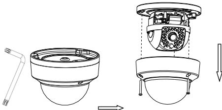
Abbildung 2-2 Kuppel abnehmen
