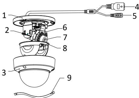
Abbildung 1-1 Kamera Übersicht
