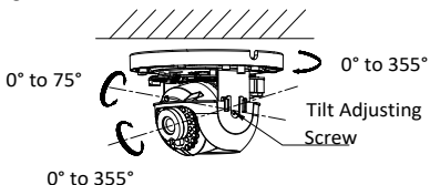
Abbildung 2-6 Kamera 3-Achsen-Einstellung
