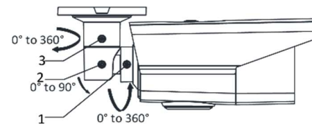
Abbildung 2-3 3-Achsausrichtung
