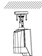
Abbildung 2-2 Kamera befestigen
