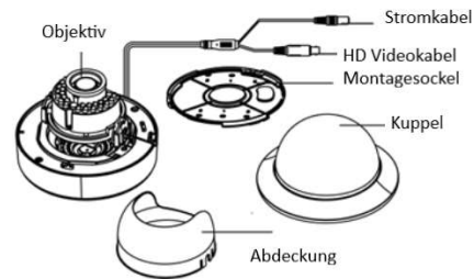
Abbildung 1-1 Kamerakomponenten
