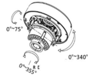
Abbildung 2-4 3-Achsenausrichtung
