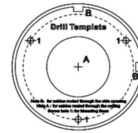
Abbildung 2-1 Bohrschablone
